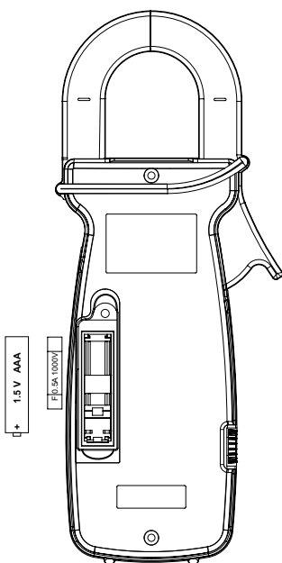
Abb. 4. Batteriesicherung
